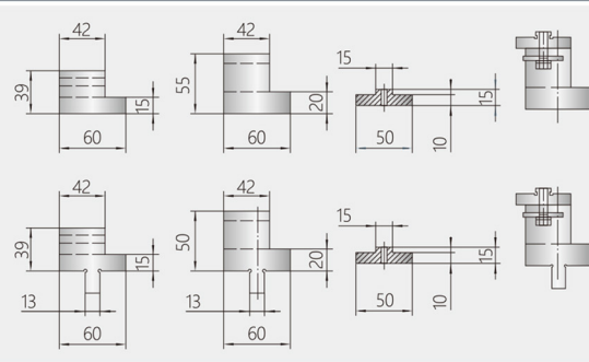
多V型下模
